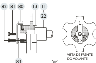
DETALHE " C " (80) MONTAGEM DA TRAVA DOS VOLANTES (80)
