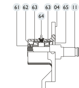
DETALHE " A " (60) MONTAGEM DO ESTICADOR DA FITA (04)
